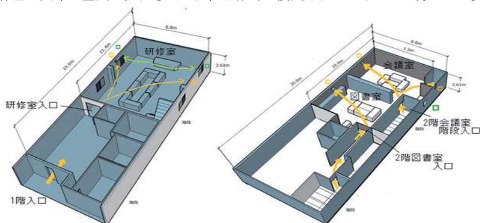
図：1階研修室（左）及び2階会議室・図書室（右）の空気の流れ
